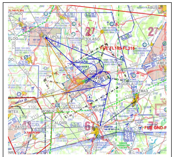
Standardverfahren IFR-Departures
